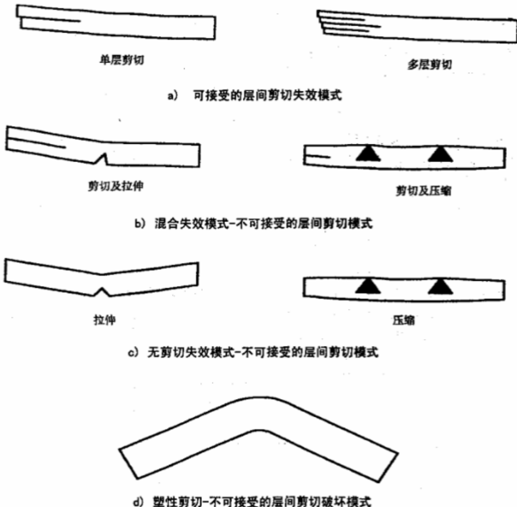
图 4 试样失效模式
