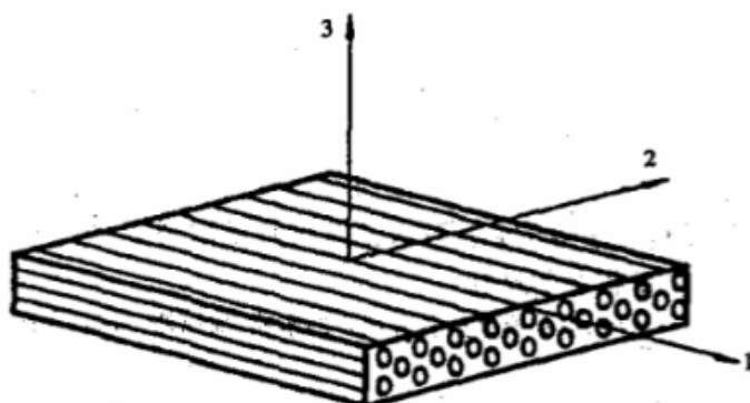
图1 单向增强复合材料板坐标轴
