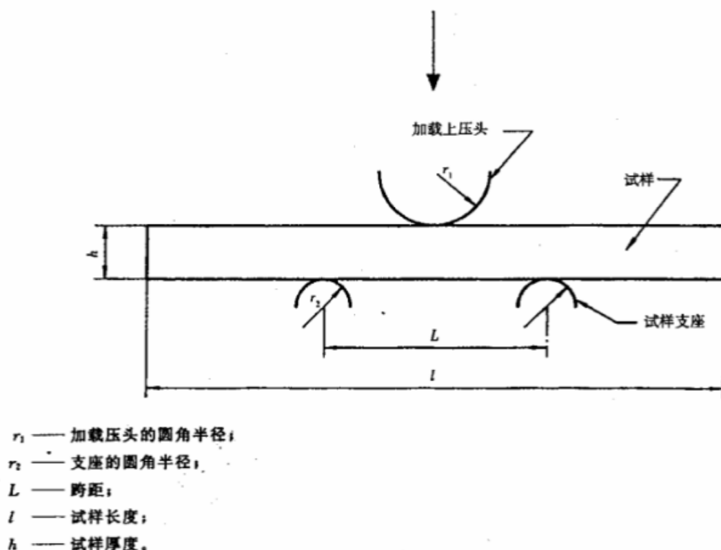
图2 加载装置
